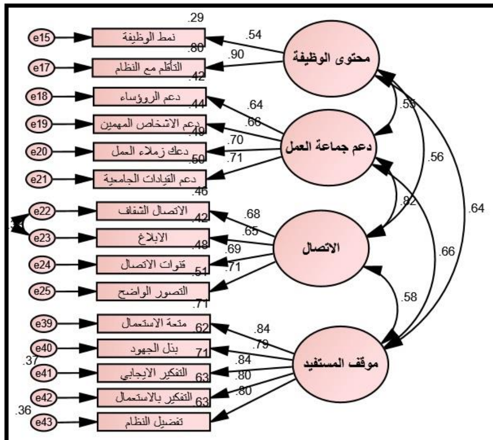
الشكل (٤): أنموذج القياس وفقاً للمستوى الأول على مستوى جميع العوامل الكامنة
