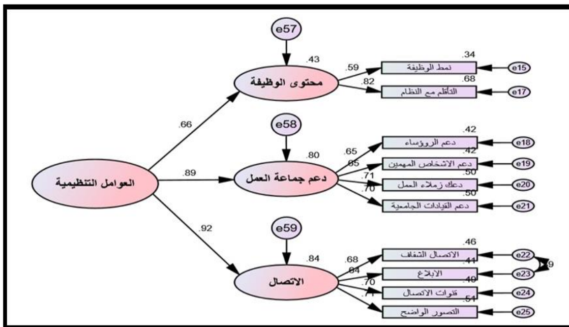
الشكل (٣): اختبار أنموذج القياس للعوامل التنظيمية وفقاً للمستوى الثاني
