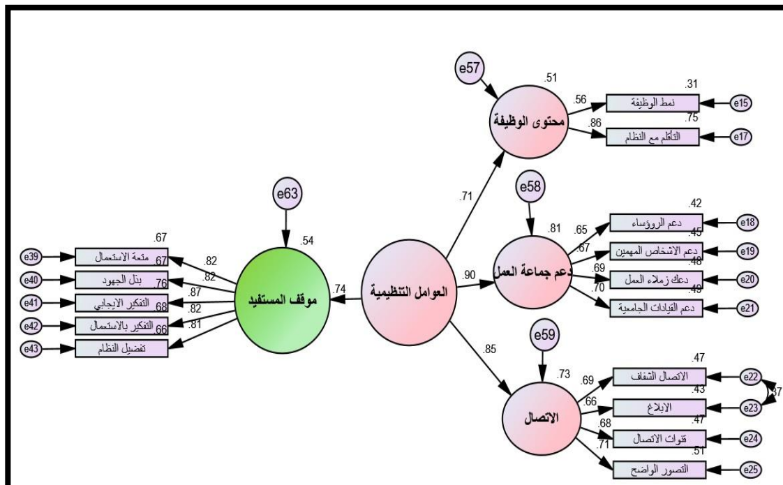
الشكل (٥): أنموذج العلاقات البنائية لتأثير العوامل التنظيمية في موقف المستفيد تجاه نظام التعليم الإلكتروني
