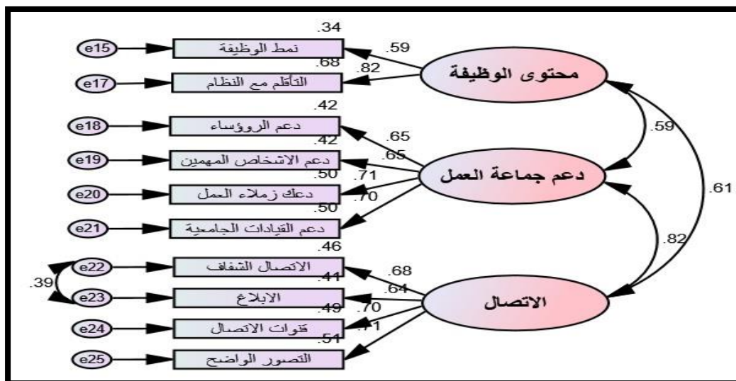
الشكل (٢): أنموذج القياس للعوامل المستقلة وفقاً للمستوى الأول في مرحلته النهائية
