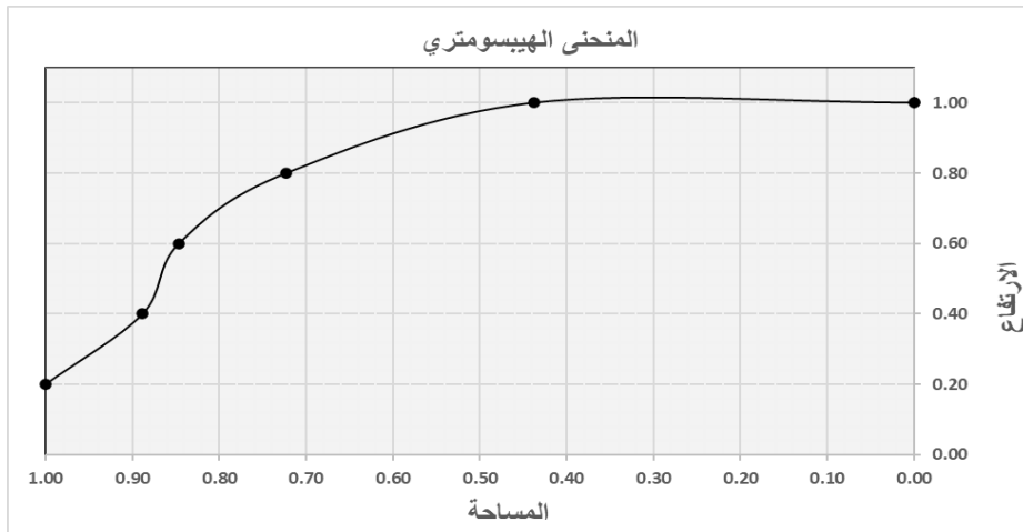
شكل (٣): المنحنى الهيسومتري لحوض حريصون
