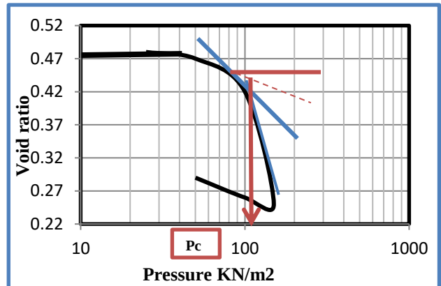
الشكل 9. العلاقة بين نسبة الفراغات والاجهاد للتربة من المحطة (3)، النموذج (C)
