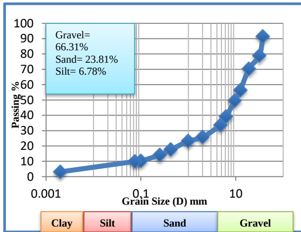
الشكل 3. التدرج الحجمي للنموذج (A2) من المحطة (1)
