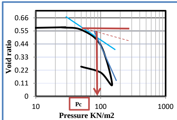
الشكل 8. العلاقة بين نسبة الفراغات والاجهاد للتربة من المحطة (1)، النموذج (A2)
