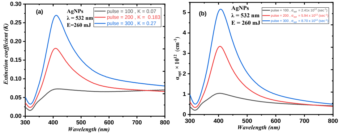
الشكل (8): (a) معامـل الخمـود ( K ), (b) الموصلية البصرية ( \sigma ) دالة للطول الموجي على التوالي ولعدد نبضات ( 100,200 and 300 ) وعند طاقة 260 mJ
