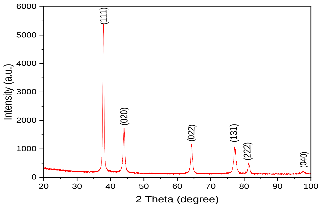
الشكل (13): حيود الاشعة السينية XRD لجسيمات الفضة
